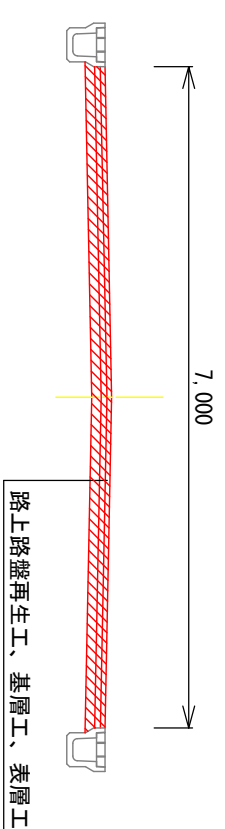
標準断面図 1:80
