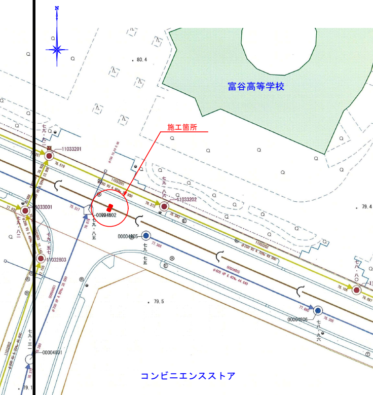
位置図 S=1:500
