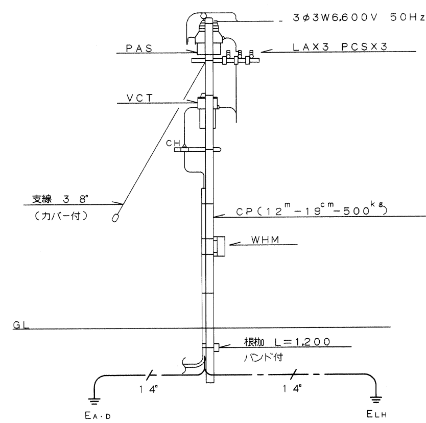
構内1号柱参考装柱図 NO SCALE
