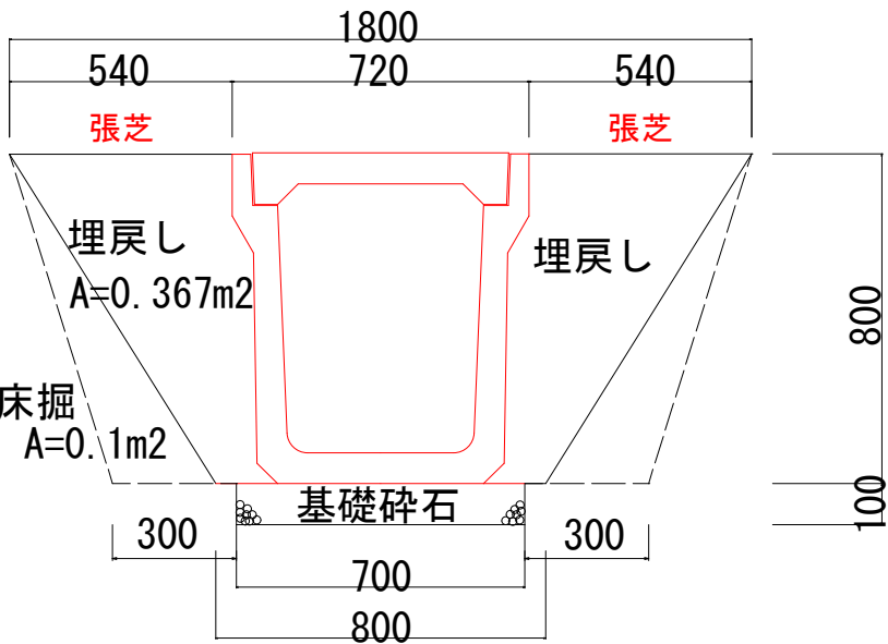
落蓋式U型側溝 500B（1：20）
