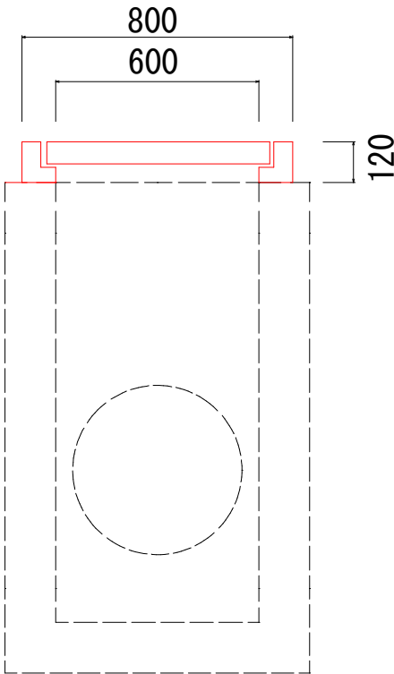
集水桧 600（G縁塊）（1：20）
