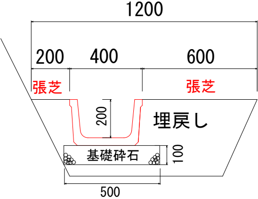
ベンチフリューム 300（1：20）
