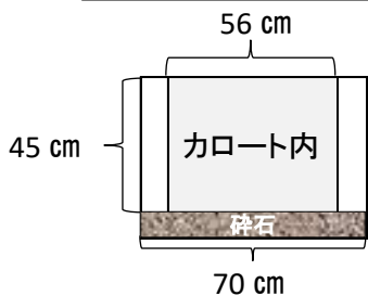
カロート断面図(正面)
