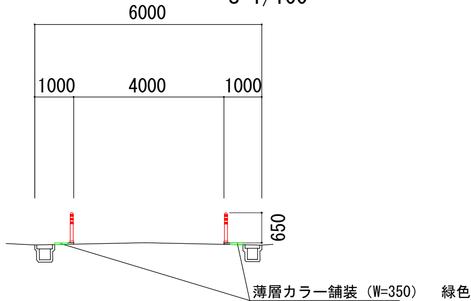
横断図
