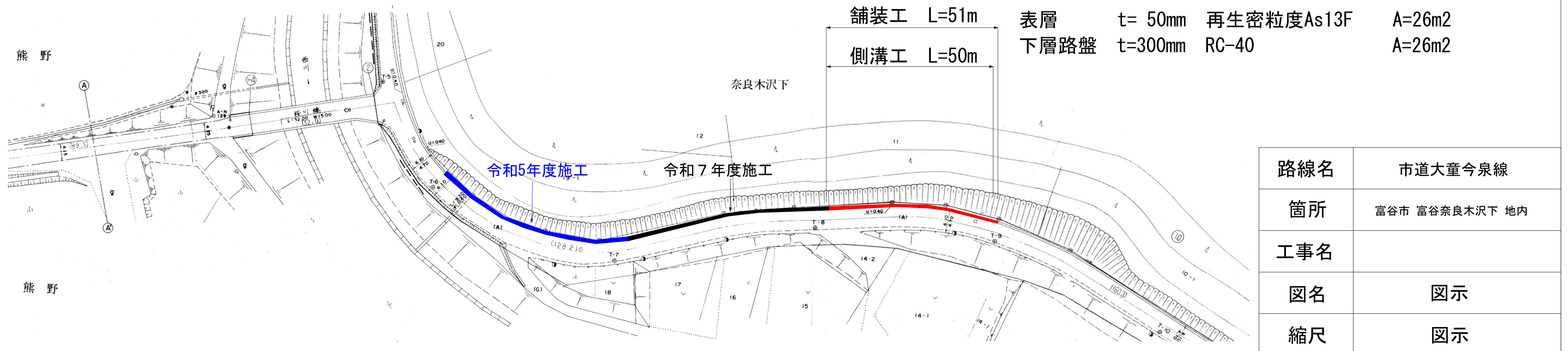
平面図 S=1/1000
