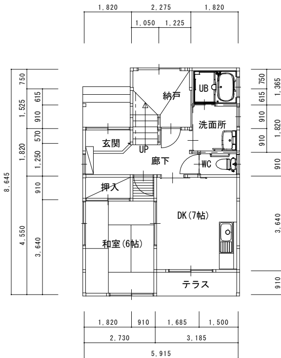
1階平面図
