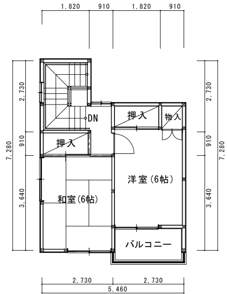
2階平面図
