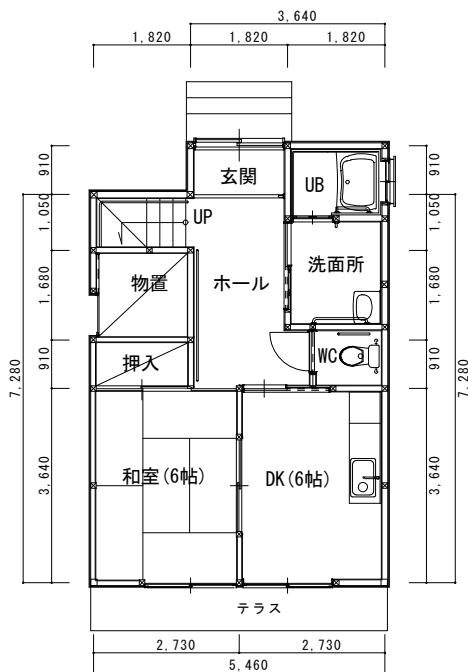
1階平面図
