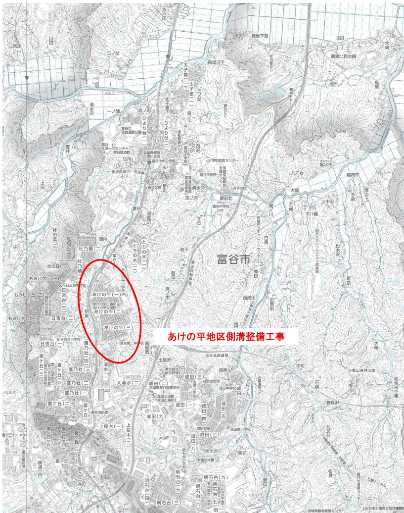
位置図
