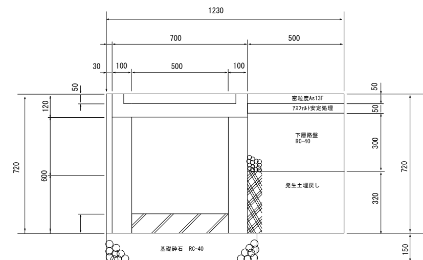
集水桮 500C (G縁塊) (1 : 20)
