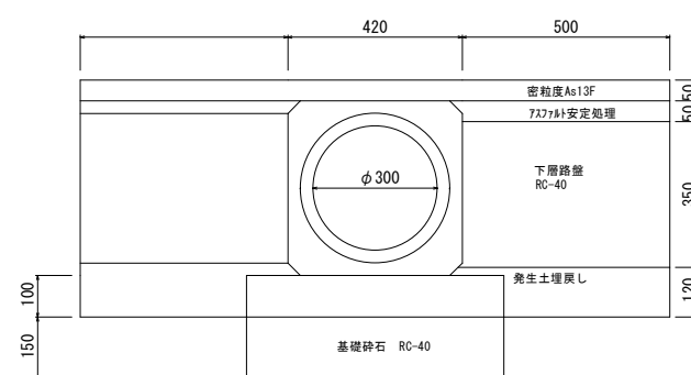
遠心ホックスカルバート CSB-1 400 (1 : 20)
