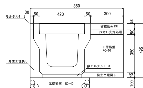
落蓋式U型側溝 3種300 (1:20)
