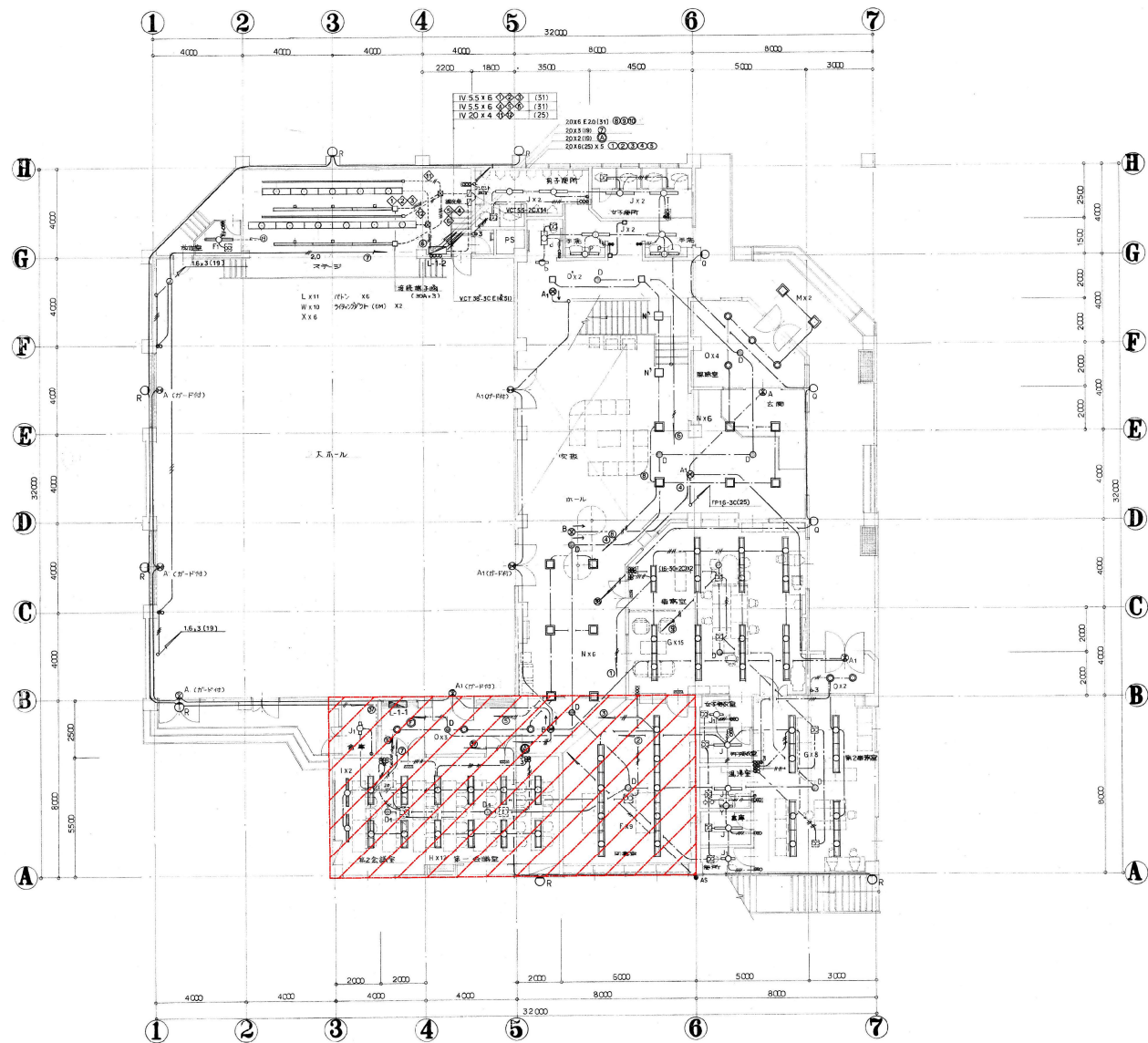
1 階平面図 1/100
