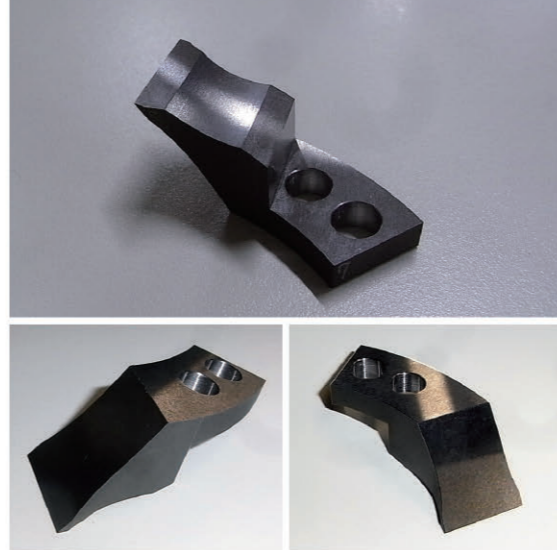
氷床掘削のドリルに使用されている刃
