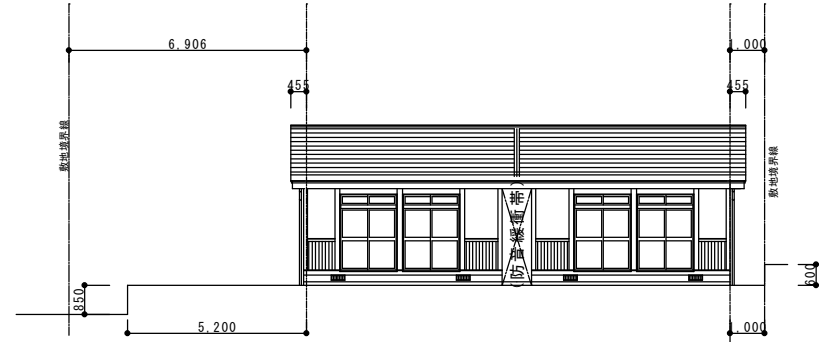
南側立面図
