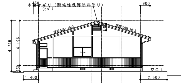
西側 立面図
