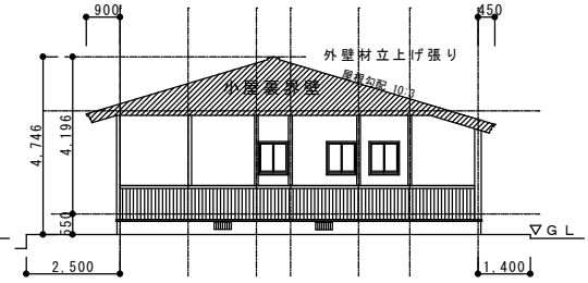
7通り東側 立面図
