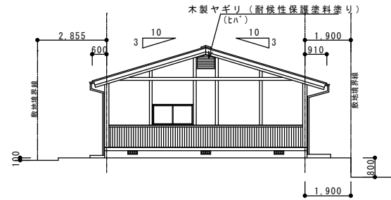
西側立面図
