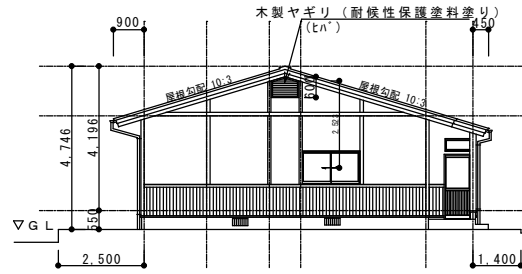
東側 立面図
