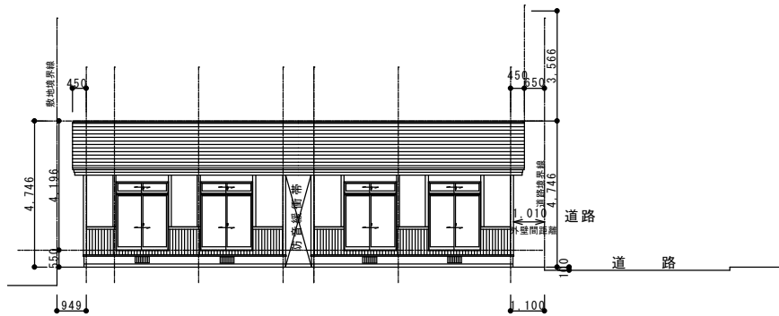
南側 立面図
