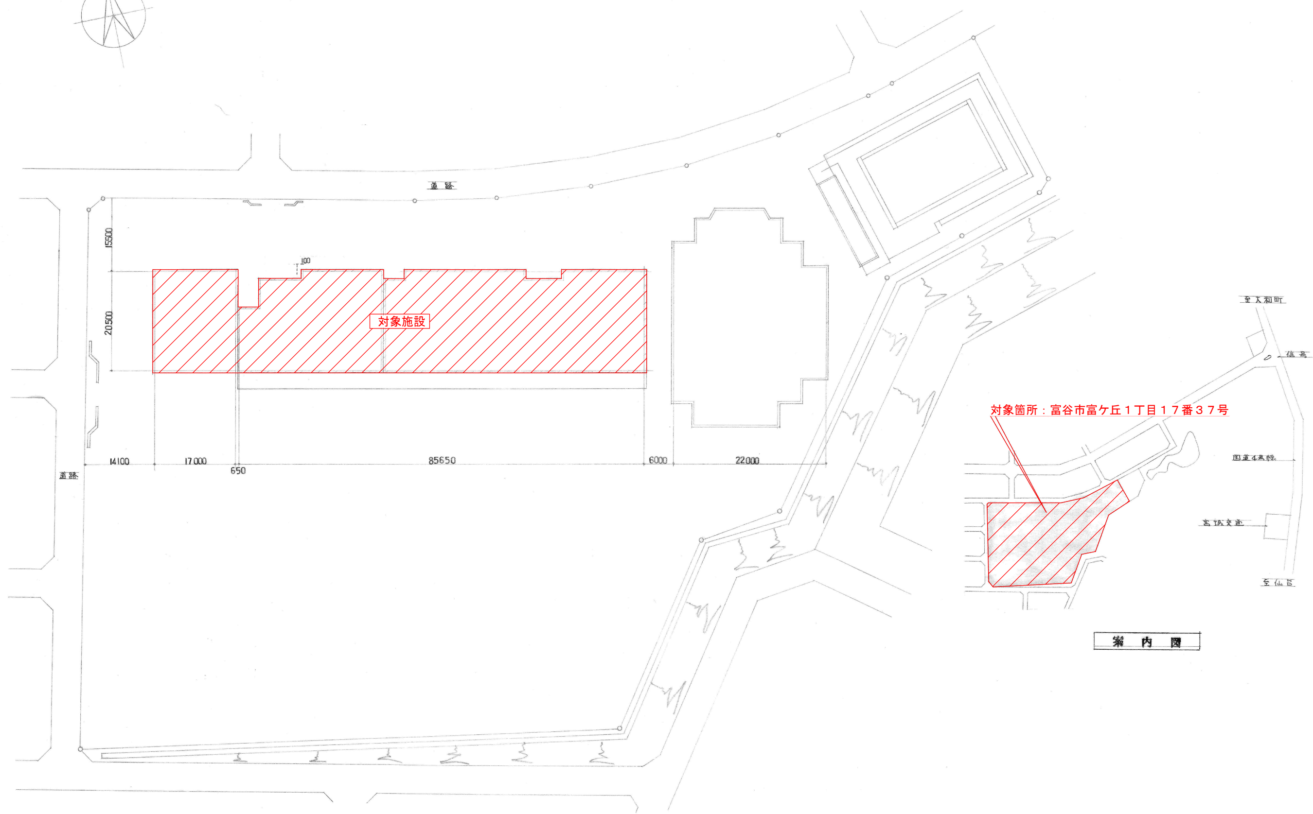
配置図 S=1:900
